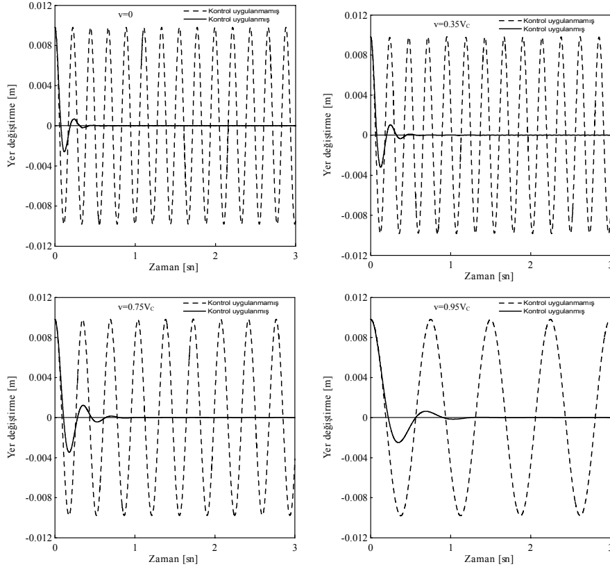
Şekil 2. Kök atama yöntemiyle tasarlanan regülatörün etkisi ( x_a=9L/16 , x_b=7L/16 )
